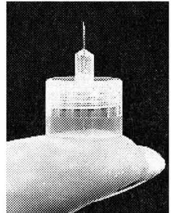
直径0.18ミリの皮下注射針。土台は直径約11ミリ＝テルモ提供
