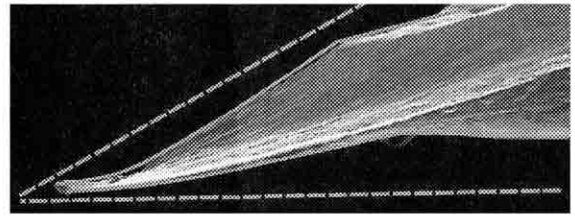
プラズマ加工は、従来の注射針（点線）よりもなめらかで鋭利な針先に加工できる＝三菱マテリアル提供
